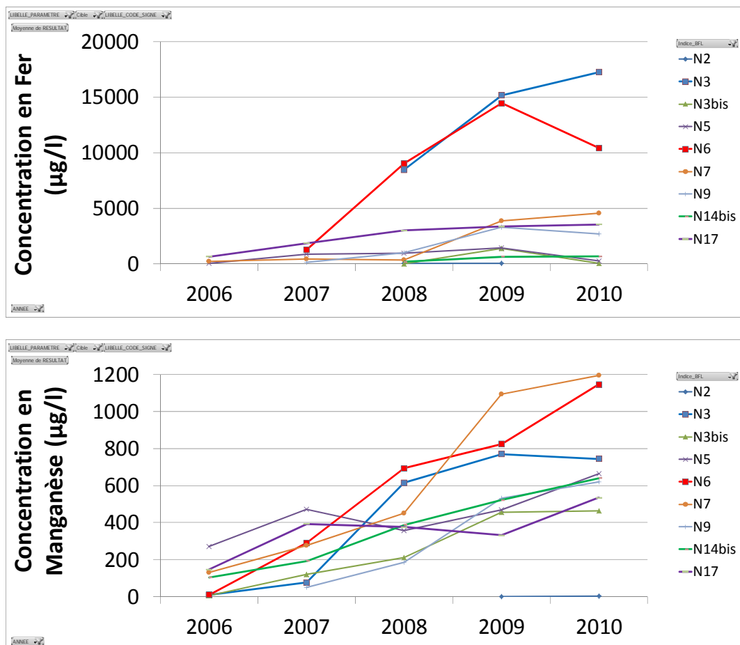
Illustration 32 : Chroniques de concentrations moyennes en fer et manganèse sur les stations du réservoir Nord
