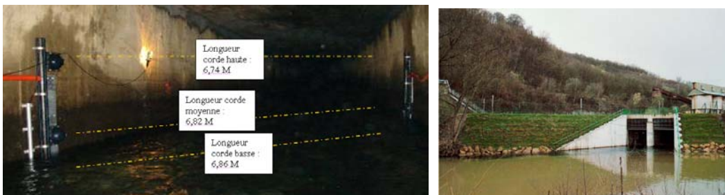
Illustration 12 : Mesure automatique du débit à la station de Moyeuve-Grande par un système « à corde » (station Kanalis)
