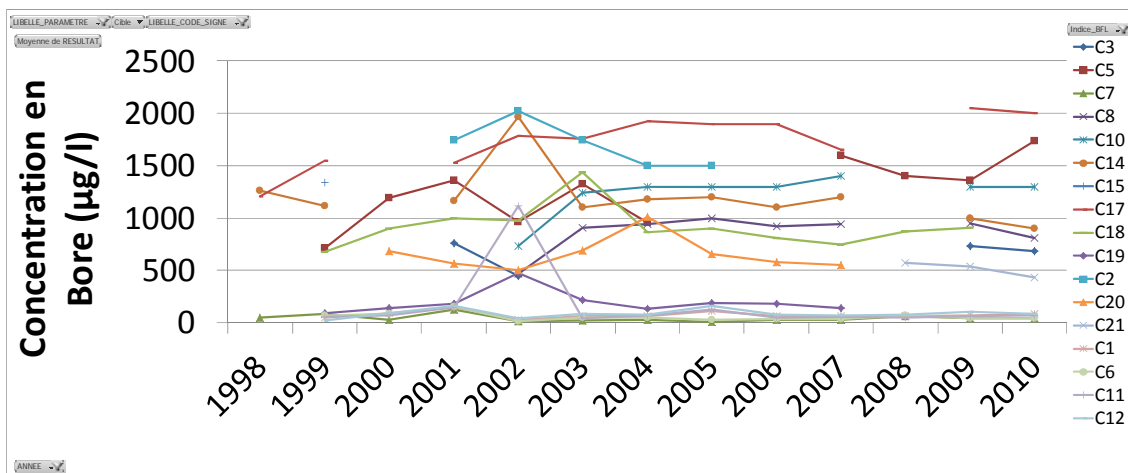
Illustration 39 : Chroniques de concentrations moyennes en Bore sur les stations du réservoir Centre
