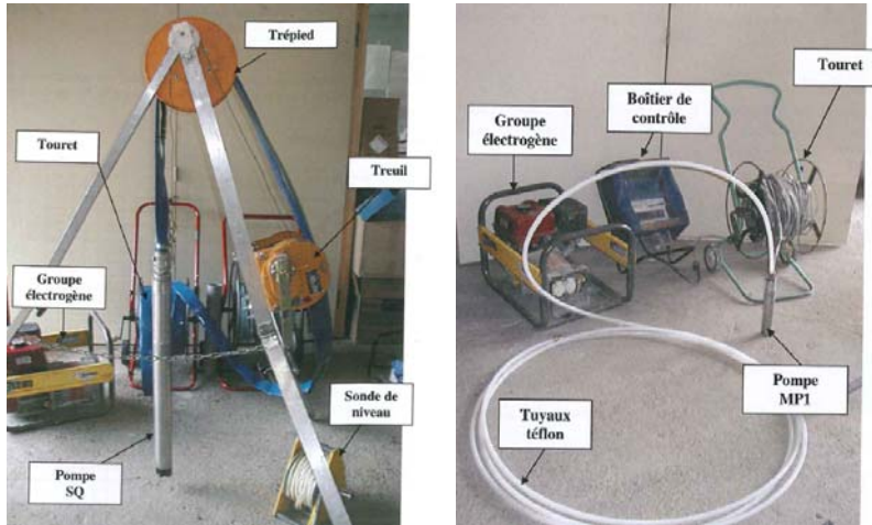
Illustration 17 : Pompes employées dans le cadre des échantillonnages (Aspect ©)
