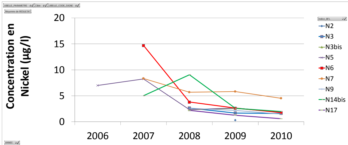
Illustration 34 : Chroniques de concentrations moyennes en nickel sur les stations du réservoir Nord
