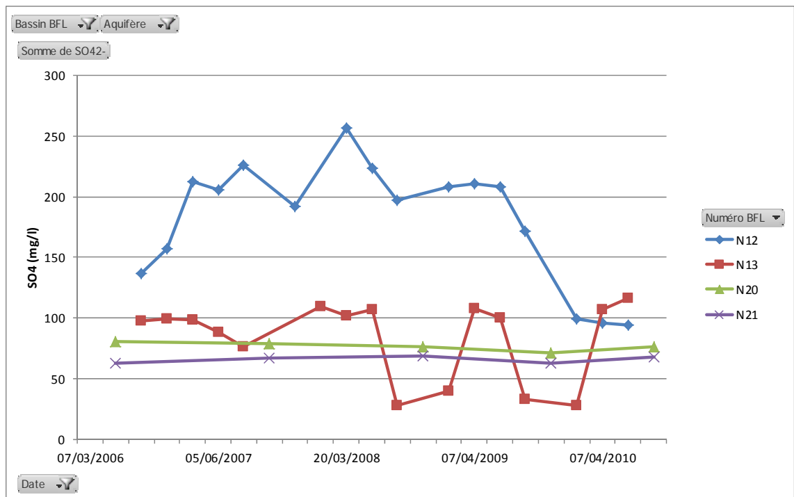
Illustration 31 : Evolution des concentrations en sulfates mesurées sur les stations implantées dans l'aquifère du Dogger du bassin Nord
