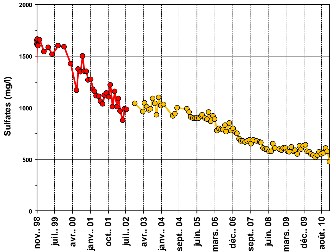
Illustration 41 : Evolution des concentrations en sulfates mesurées sur le point de débordement du réservoir Sud (la courbe rouge correspond aux mesures effectuées sur l'ancien point de débordement de la galerie du tunnel de Moyeuivre)
