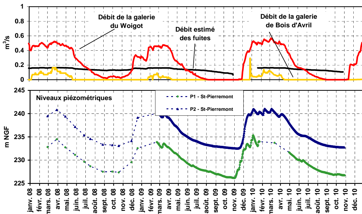
Illustration 23 : Débit de débordement en m 3 /s du réservoir centre
