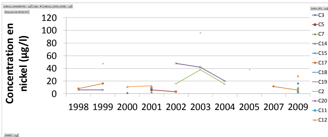
Illustration 40 : Chroniques de concentrations moyennes en Nickel sur les stations du réservoir Centre
