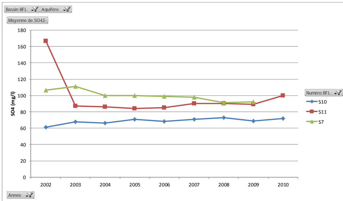
Illustration 42 : Evolution des concentrations en sulfates mesurées sur les stations implantées dans la formation ferrifère non exploitée
