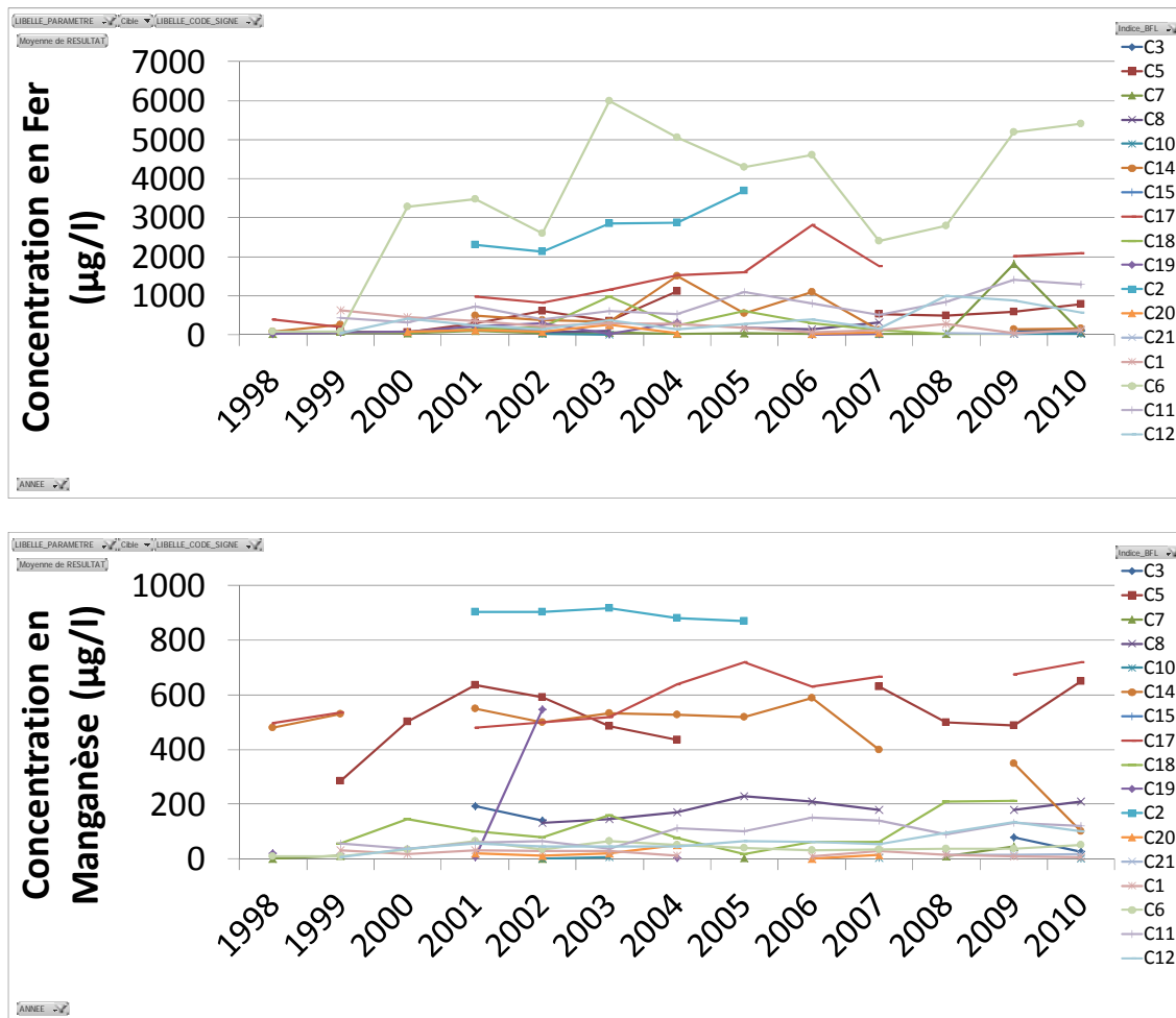
Illustration 38 : Chroniques de concentrations moyennes en fer et manganèse sur les stations du réservoir Centre
