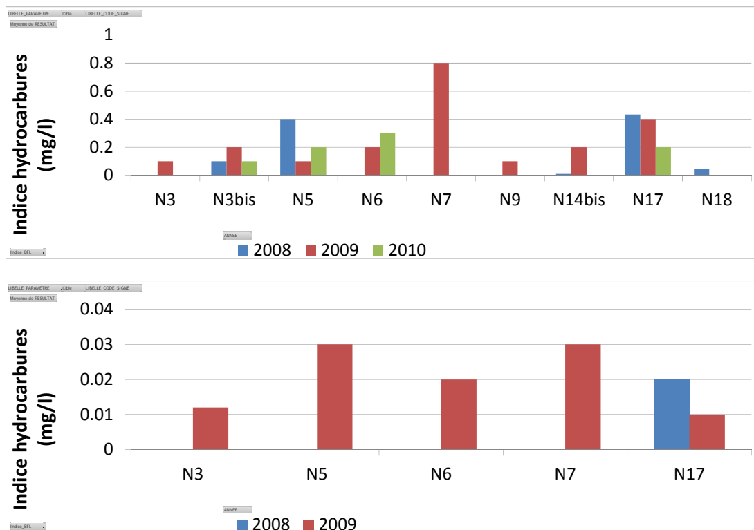
Illustration 35 : Maximums annuels des teneurs en indice hydrocarbures et phénols
