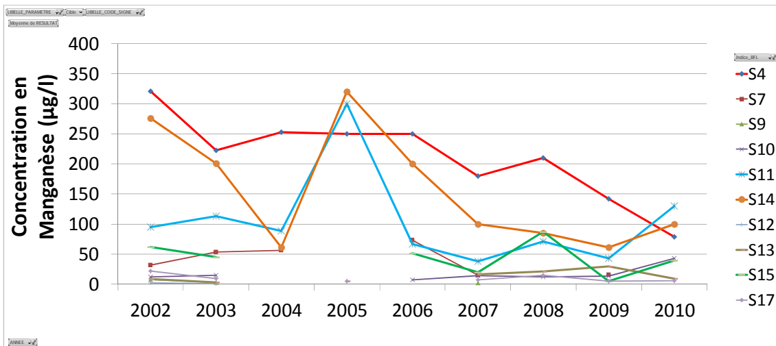
Illustration 45 : Chroniques de concentrations moyennes en manganèse sur les stations du réservoir Sud
