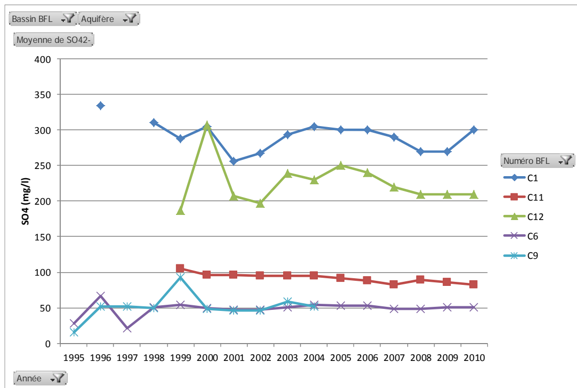
Illustration 37 : Evolution des concentrations moyennes annuelles en sulfates mesurées sur les stations implantées dans l'aquifère du Dogger du bassin Centre
