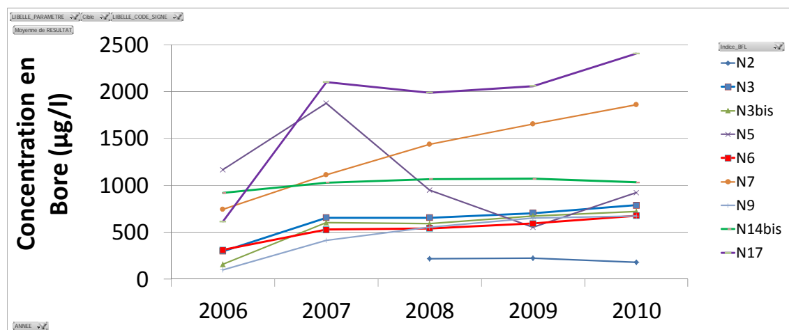
Illustration 33 : Chroniques de concentrations moyennes en Bore sur les stations du réservoir Nord
