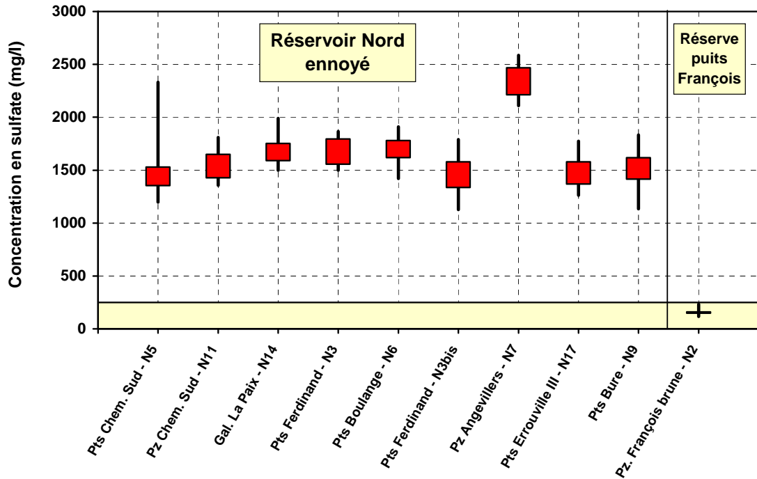
Illustration 29 : Diagramme type « boîte à moustaches » des concentrations en sulfates sur les stations du réservoir Nord
