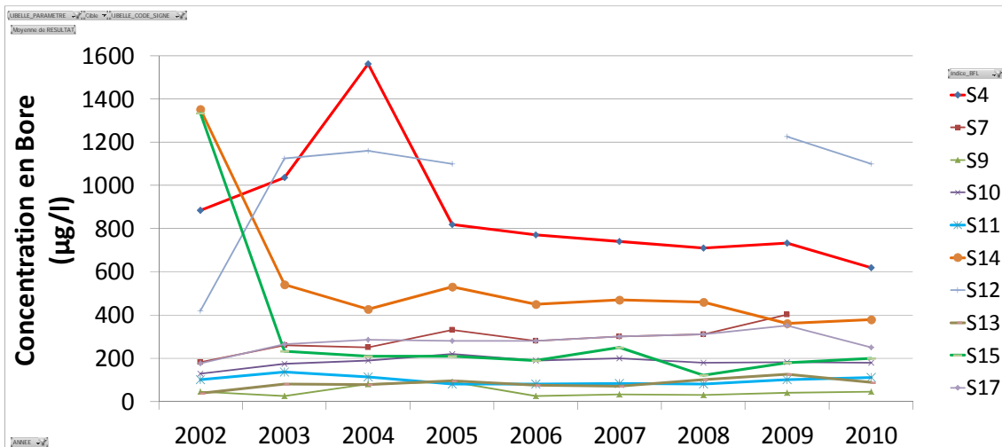
Illustration 46 : Chroniques de concentrations moyennes en bore sur les stations du réservoir Sud
